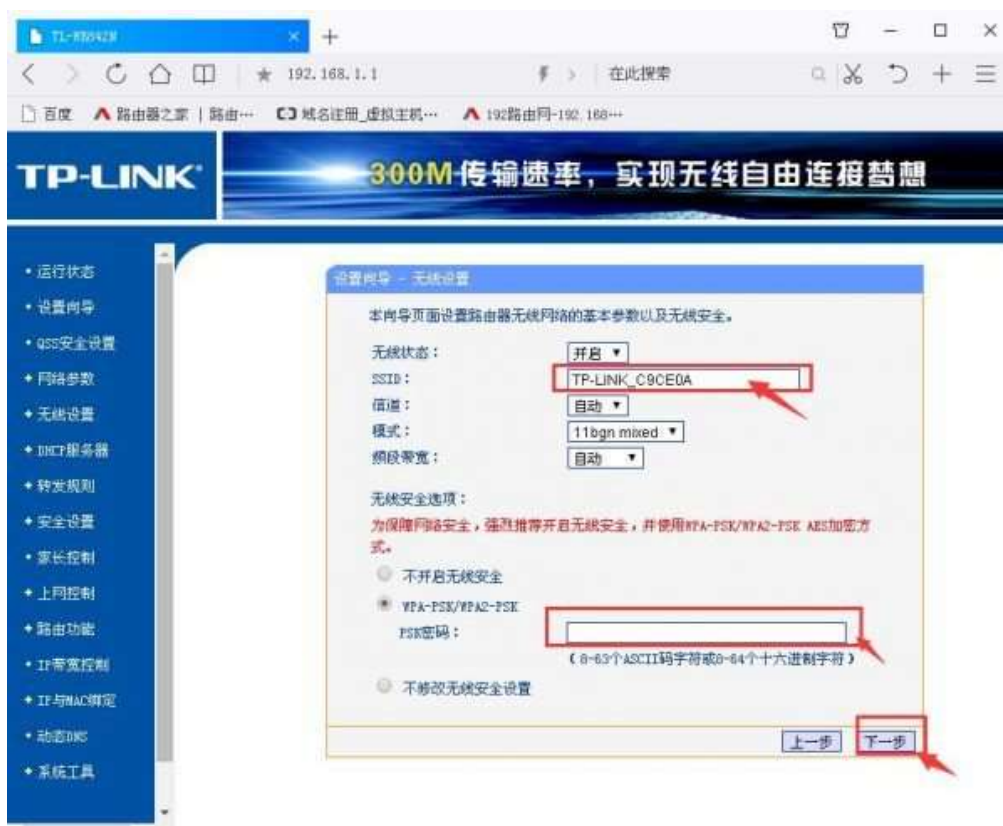
图 3 设置密码
